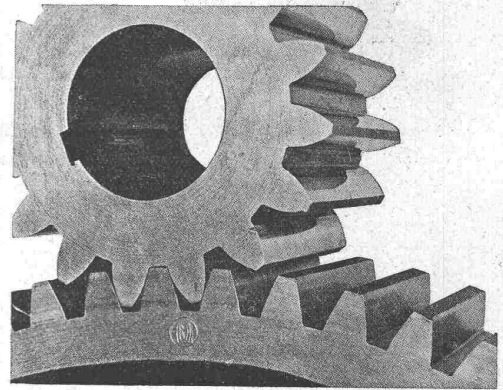
Figur 4. Mit gehärtetem und geschliffenem Maag-Ritzel.
