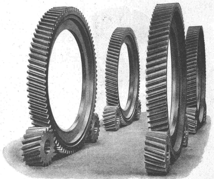
Figur 6. Triebrädersatz für eine elektrische Vollbahnlokomotive. Gehobelte Maag-Verzahnung.
