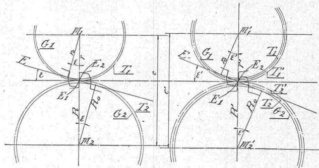
Figur 1. Evolventenverzahnung.
