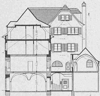
Abb. 6. Schnitt. — Masstab 1:400.
