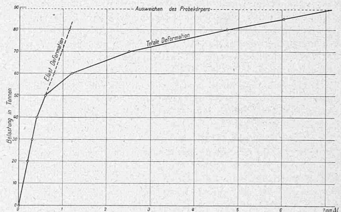
Abb. 3. Diagramme der Druckproben-Ergebnisse.
