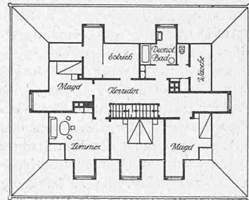
Abb. 2. I. Stock. Abb. 3. Dachstock. Masstab 1 : 400.
