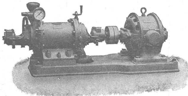
Kesselspeise-Zentrifugalpumpe
