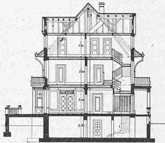
Abb. 2 bis 4 Grundrisse, Abb. 5 Schnitt zur Villa Arbenz. — 1 : 400.
