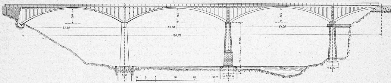
Abb. 10. Brücke über die Rhone bei Puyon, unterhalb Bellegarde, erbaut 1906/1907. — Längsschnitt und Ansicht, etwa 1:1000.
