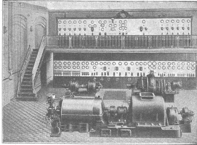
Schaltwand in der Werkzentrale der Nähmaschinenfabrik Singer in Podoisk (Russland).
