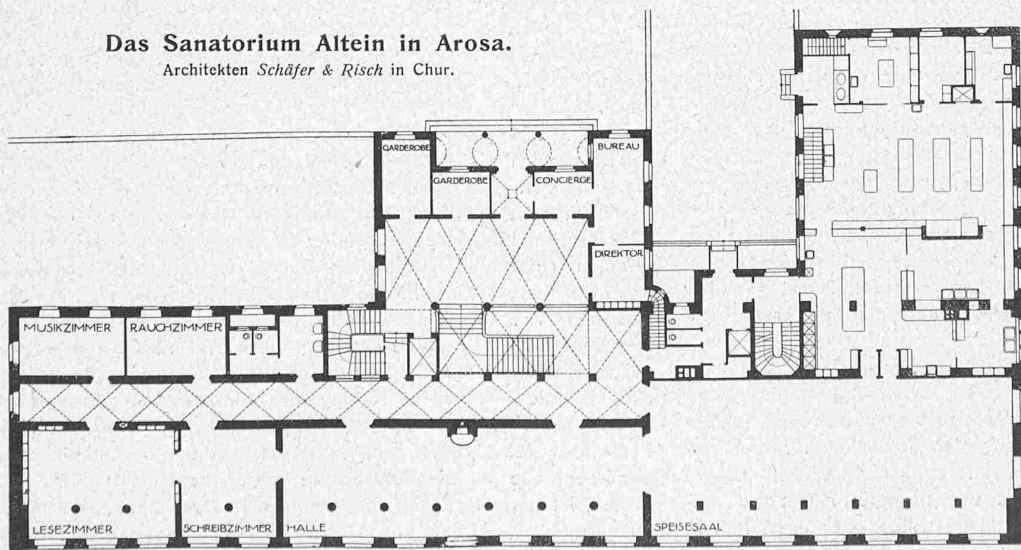
Abb. 2. Grundriss vom Erdgeschoss (Obergeschoss vergl. S. 78). — Masstab 1:450.
