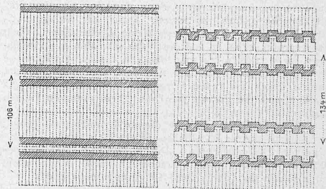
Abb. 1. Schema von Reihenhau (links) und Gruppenbau (rechts) 1:5000 mit je 40 m 2 überbauter Fläche und 200 m 2 Gartenland pro Grundstück.
