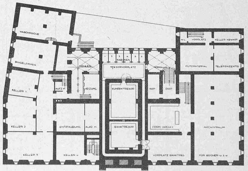
II. Preis, Entwurf Nr. 17. — Arch. Gebr. Pfister, Zürich. — Keller, Erdgeschoss, I. Stock. — 1 : 500.
