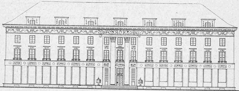
Fassade an der Bahnhofstrasse und (darunter) Schnitt. — Masstab 1 : 500.
