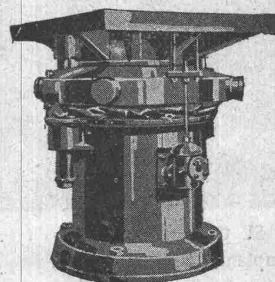
Stossfreie Rüttelformmaschine D. R. P.
