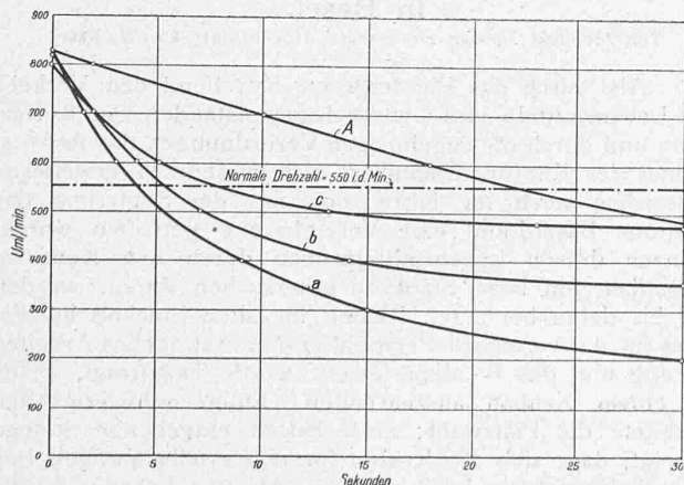
Abb. 4. Vorversuche über die Wirkung der Streustrahlen.
