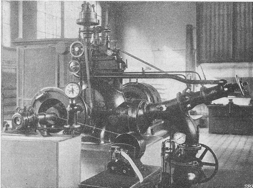
Abb. 6. Versuchs-Anordnung im Maschinen-Laboratorium der Eidg. Techn. Hochschule.
