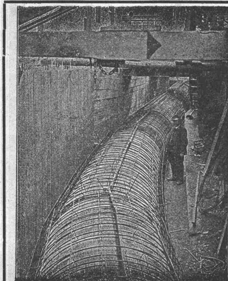
Druckrohr in Eisenbeton von 2 m Durchmesser der Wasserkraftanlage Stöcklin & Cie., Basel, 1916/17.
