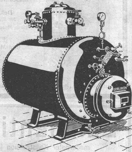
Röhrendampfkessel 120 kW
