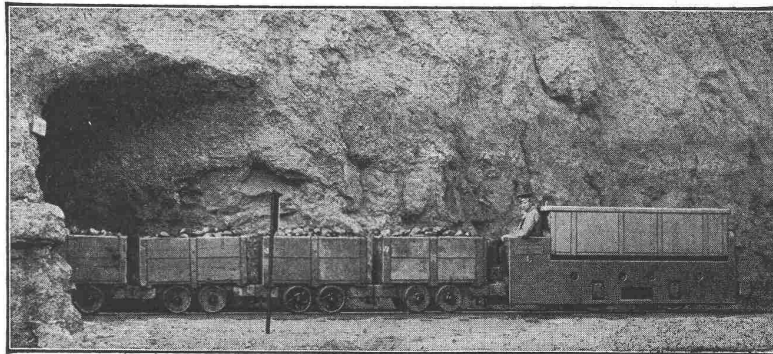
Grubenbahn Gr. Bülden, mit abrollbarer Batterie
