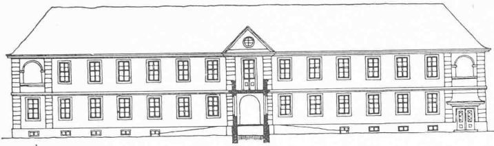
Südfrent 1:500.
