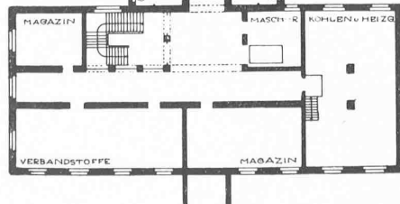
Grundrisse vom Untergeschoss, Erdgeschoss, I. Stock und Dachgeschoss. — 1:500.
