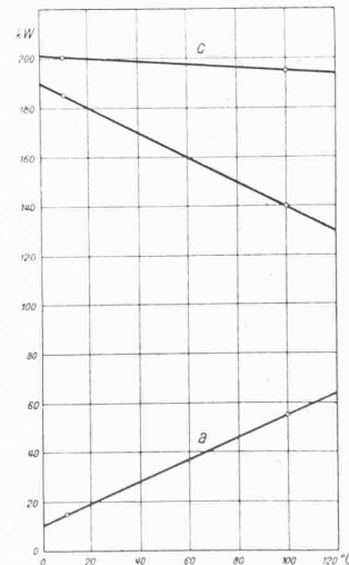
Abb. 6. Leistung eines Warmwasser-Kessels mit kombinierten Widerständen. a Leistung durch das Wasser, b Leistung durch den Eisendraht, c Gesamtleistung.
