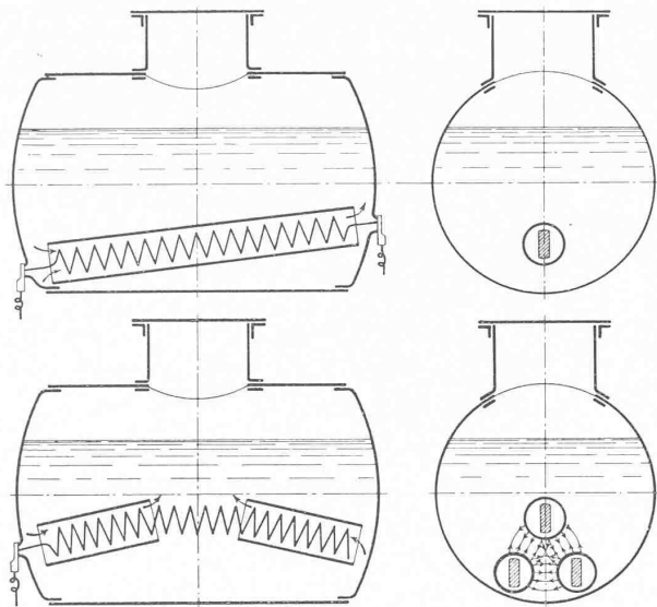
Abb. 3 und 4. Kessel mit wasserberührter Widerstandsheizung, oben mit Stromdurchgang nur durch den Draht, unten mit Stromdurchgang teils durch den Draht, teils durch das Wasser.
