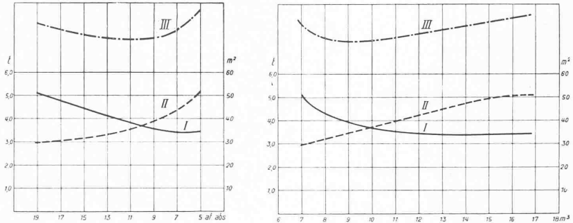
Abb. 12 und 13. Veränderlichkeit des Eisengewichts des leeren Speichers (I) und der Speicher Oberfläche (II) mit dem Ladedruck (Abb. 12) bzw. mit dem Speicherinhalt (Abb. 13) für eine Dampfentnahme von 1000 kg bei einem Entladedruck von 2 at.
