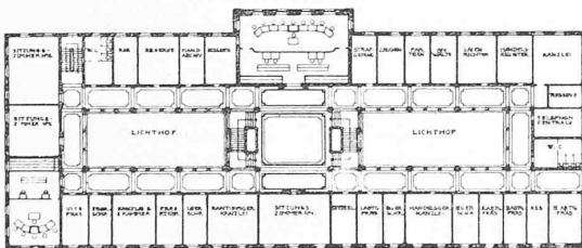
Grundrisse vom II. und III. Stock. — 1 : 1000.
