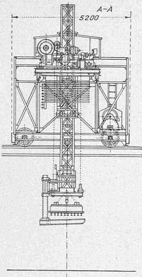
Abb. 3. Seitenansicht der Laufkatze mit Hubwerk. Masstab 1 : 150.
