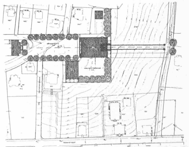
Zum Wettbewerb für die Reform. Kirche Arbon. — Entwurf Nr. 39 (in enger Wahl). Lagepläne von Arbon 1:15 000 und von der Baustelle 1:2500.
