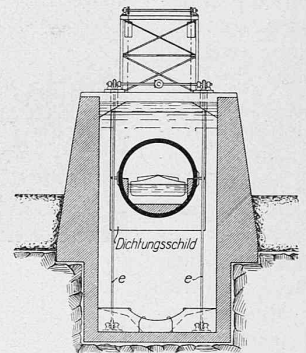
Abb. 2. Querschnitt der Schleuse.
