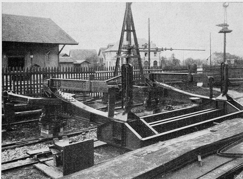
Abb. 5. Ueberblick auf die Spannvorrichtung; vorn der Gewichtsklotz-Träger.
