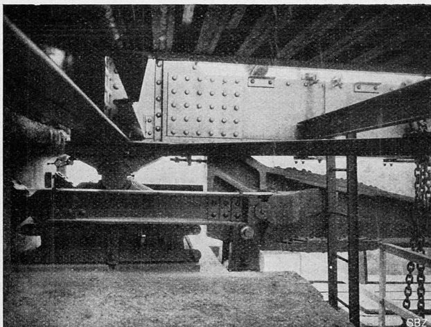
Abb. 7. Uebertragung der Hebelkraft am beweglichen Auflager auf Pfeiler 10.
