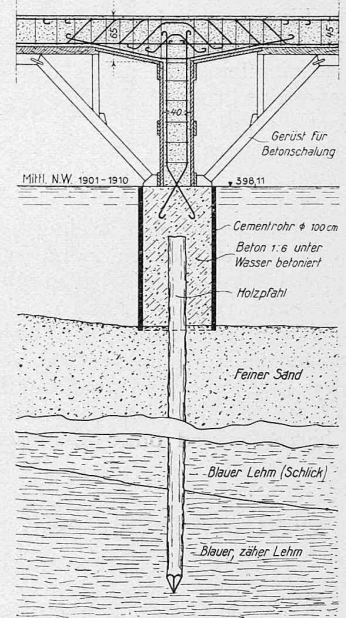
Unterbau-Konstruktion. — 1 : 100.
