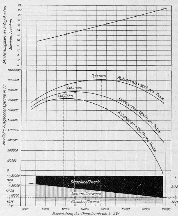
Abb. 8. Ersparnis an Anlagekapitel und Jahresausgaben bei Deckung des Energiebedarfs gemäss Abb. 7 unter Mitnwendung von Dieselmotoren anstatt gemäss Abb. 6 durch reine Wasserkraft.
