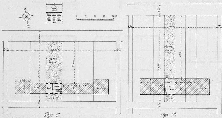
Abb. 13. Schematischer Vergleich der Grundriss-Typen A und B. — Masstab 1:1000. Architekten Kölla & Roth, Wädenswil.
