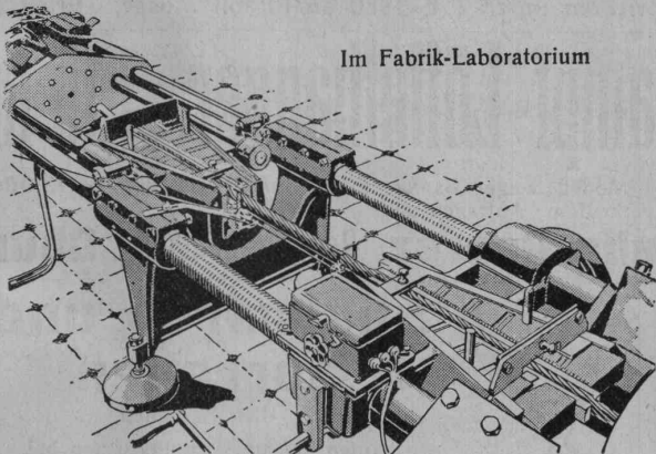
Drahtseil-Zerreiss-Versuch
