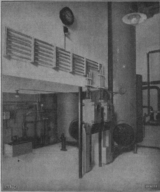
ELEKTRISCHE WARMWASSER-BEREITUNGS-ANLAGE IN DER KRANKEN-ANSTALT AARAU LEISTUNGS-AUFNAHME PRO APPARAT 80 kW
