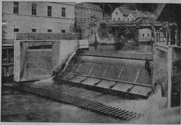
Dachwehr in der Mürz der Kabelwerke Felten & Guilleaume, Bruck a. d. Mur.
