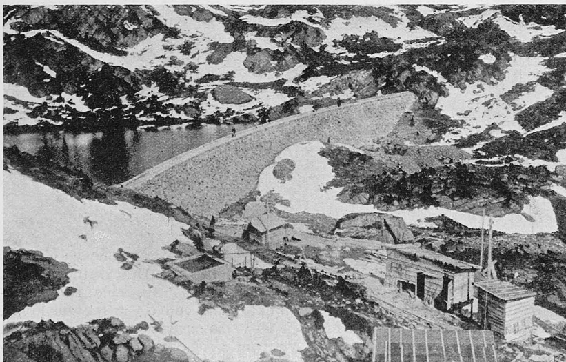
Abb. 7. Die Stauauer am Fully-See nach deren Fertigstellung bis auf Kote 2137,0.
