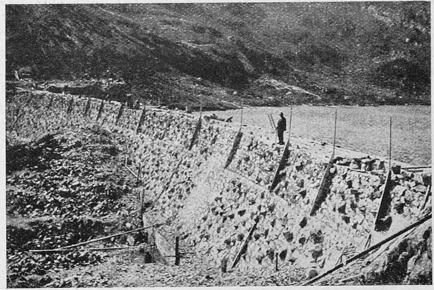
Abb. 6. Die Stauauer während der Bauarbeiten.
