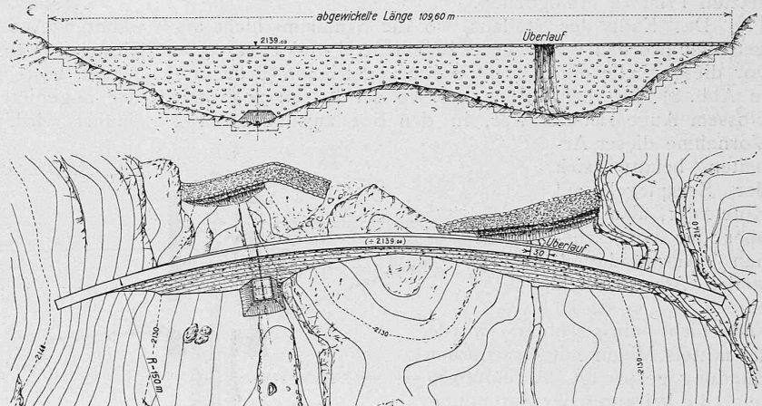
Abb. 4. Grundriss und Aufriss der Stauauer nach ihrer Erhöhung auf Kote 2139. — Masstab 1:1000.
