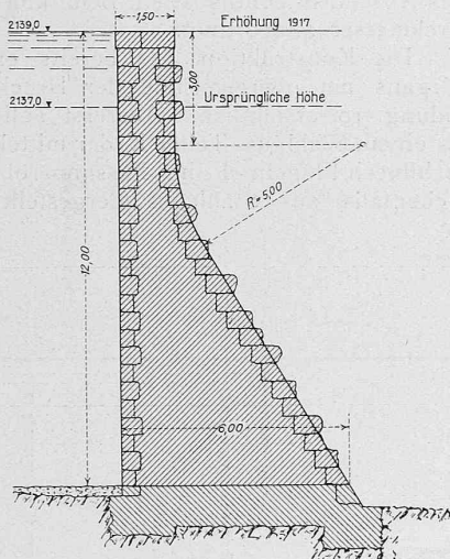
Abb. 5. Querschnitt durch die Stauauer. — 1:200.
