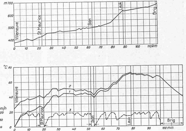
Abb. 9. Vorausberechnete mittlere Erwärmung der Motor-Rotoren auf der Strecke Villeneuve-Brig. Kurve 1 bei der ersten, Kurve 2 bei der zweiten Bergfahrt, bei Fahrgeschwindigkeiten nach Kurve 3. Darüber das Längenprofil.
