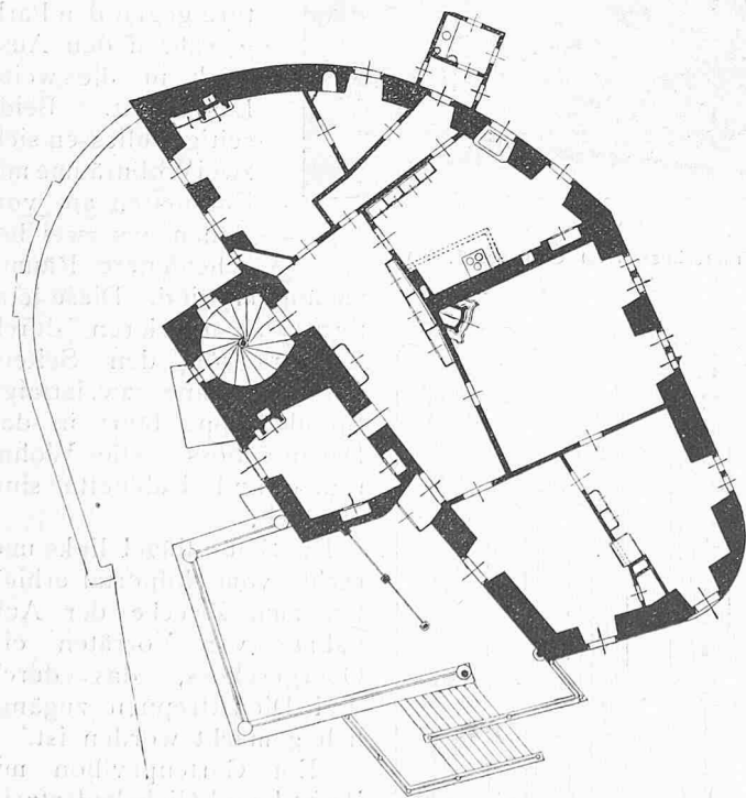
Grundriss des Kellers.
