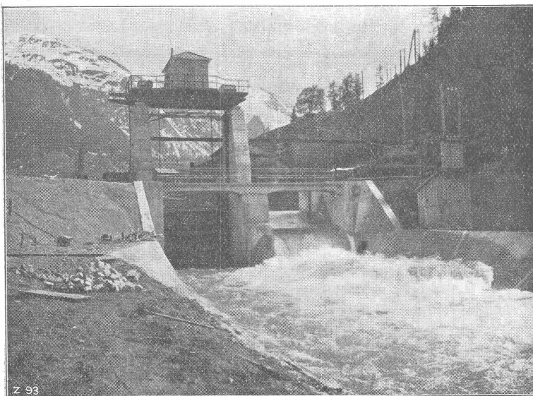
Wasserrfassung des Kraftwerkes Klosters-Küblis Ausgeführt 1920/21
