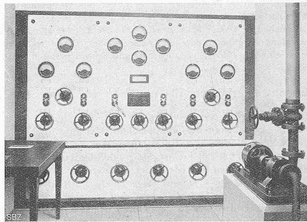
Abb. 2 und 3. Regulierzimmer. Links die beiden 4 PS Zirkulationspumpen, rechts die 0,7 PS Zirkulationspumpe für den Sommerbetrieb.
