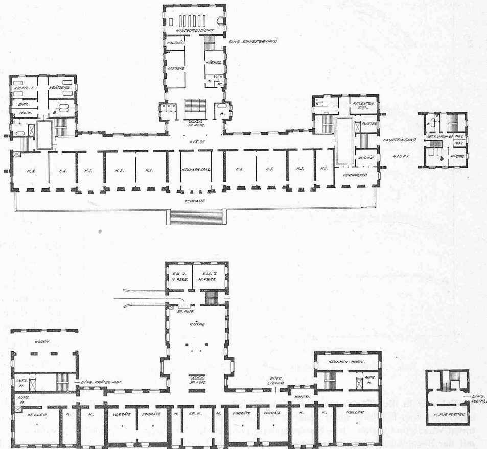
Grundrisse vom Kellergeschoss, vom Erdgeschoss und vom ersten Obergeschoss. — Masstab 1:800.
