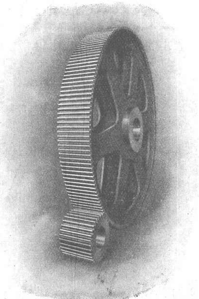
Stirnrad-Getriebe mit gehärtetem und geschliffenem Ritzel für Förder-Anlage 1100 PS.
