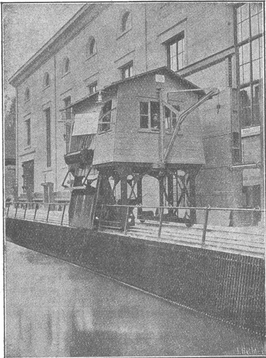
ELEKTRIZITÄTSWERK WYNAU-LANGENTHAL Kombinierte Rechen-Reinigungsmaschine mit doppeltem Schwenkran
