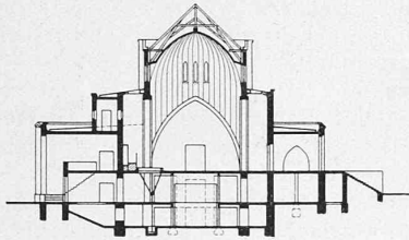
Abbildung 10. Längsschnitt.
