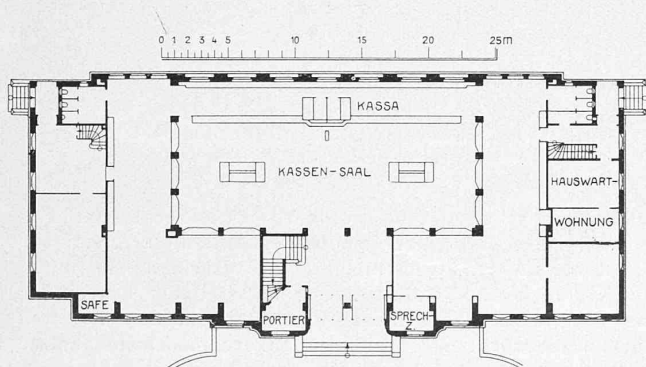
Abb. 5. Oesterreichisches Verkehrsbureau. Erdgeschoss-Grundriss 1:500.
