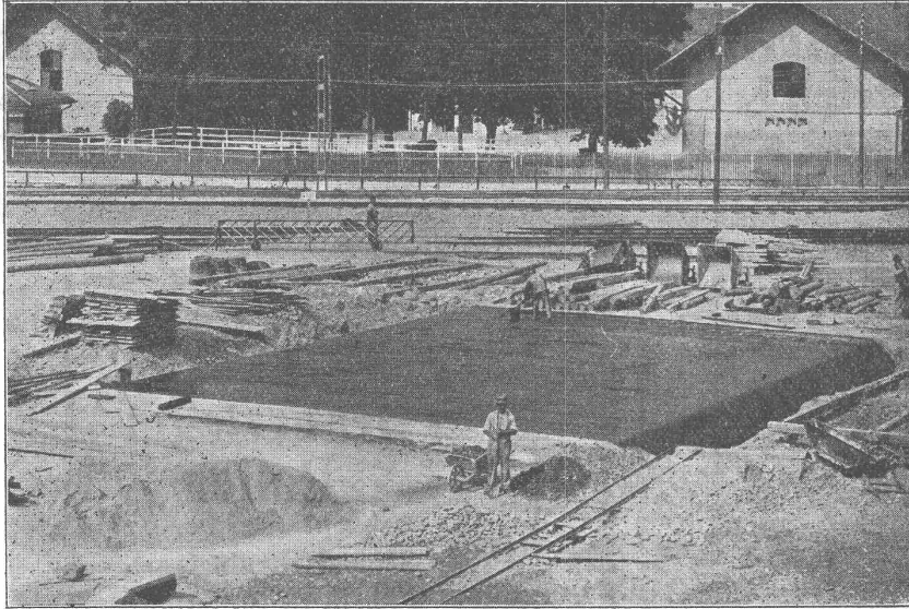
Mittlerestrasse-Unterführung Thun S. B. B. Mammut-Isolierung ausgeführt durch Asphalt- Bau-Unternehmung H. Tschaggeny, Thun. Emulsion A.-G., Zürich.
