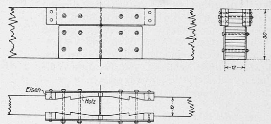
Abb. 10. Stossverbindung nach Vorschlag Hübner.
