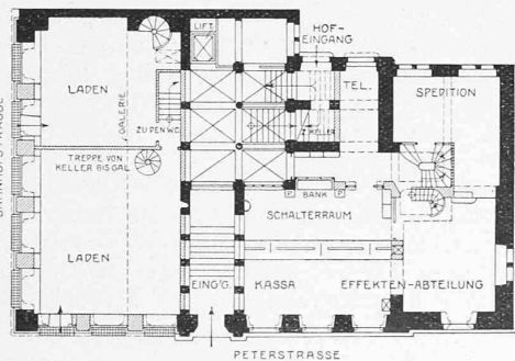
Entwurf „Lasius“. Schnitt und Grundrisse vom Erdgeschoss und 1. Stock. Masstab 1 : 400.
