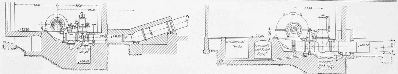
Abb. 9 und 10. Querschnitte durch das Maschinenhaus; links eine der beiden 4000 PS-Turbinen, rechts die 12000 PS-Turbine. — Masstab 1 : 250.
