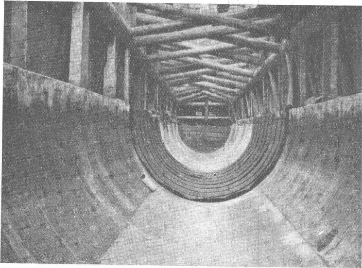
Bündnerische Kraftwerke A.-G.: Heberleitung in Klosters (330 m lang) Baulitung: R. Moor, Ingenieurbureau, Zürich Wasser- und luftdichte Isolation des Heber- Unternehmung: Locher & Co., Zürich rohrtes mit „Mammut“ . . . . . 3000 m 2 Ausgeführt durch Asphalt-Emulsion A.-G.
