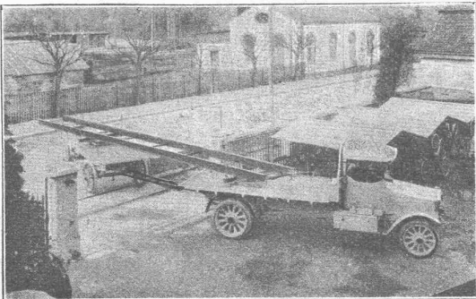
Berna 5-Tonnen mit Anhänger für Betoneisentransport
