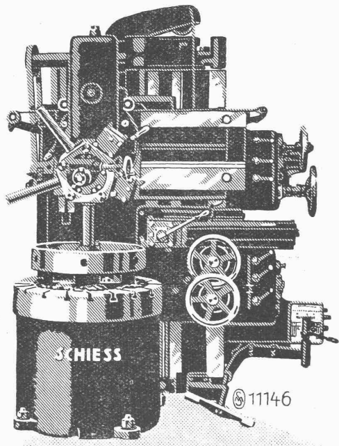
Einständer-Karussell mit 1250 mm Drehdurchmesser zur wirtschaftlichen Bearbeitung von Massenteilen aller Art.
