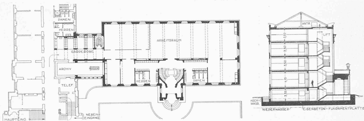
Abb. 2. Grundriss des Erweiterungsbaues (links Anschluss an den bestehenden Bau). — Masstab 1:500. — Abb. 3. Schnitt.
