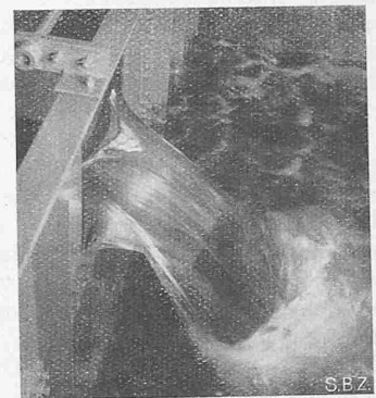
Abb. 13. Ueberfallwehr, hergerichtet für Ueberfall mit Seitenkontraktion.
