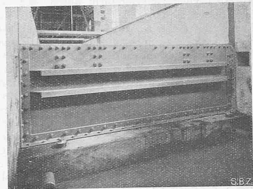
Abb. 12. Ueberfallwehr, hergerichtet für Ueberfall ohne Seitenkontraktion.
