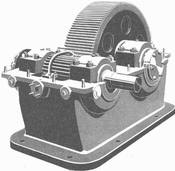
Ritzel mit gehärteten und geschliffenen Zähnen Rad mit gehobelten Zähnen 16 Getriebe an eine Zementfabrik in Belgien geliefert
