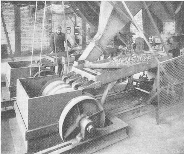
Abb. 2. Elektromagnetischer Aschenscheider, System Ullrich.
