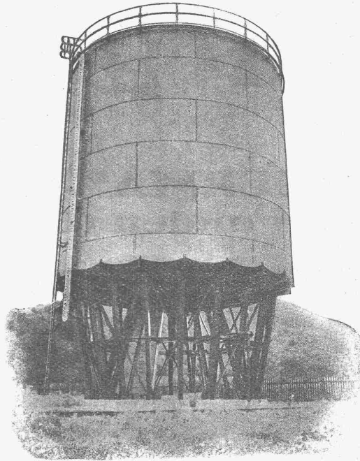
Genieteter Laugenbehälter von 1000 m 3 bzw. 1350 Tönnen Inhalt, 10,8 m Durchmesser, 12 m Höhe, mit Spezialbodenkonstruktion.
