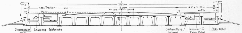
Abb. 33. Querschnitt der Brücke für die Badenerstrasse (schwerster Träger 8,2 t).
