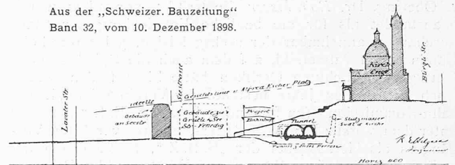
Abb. 1. Bahnhof Engen an der Grütlstr., nach Projekt Hilgard. — 1 : 2000.
