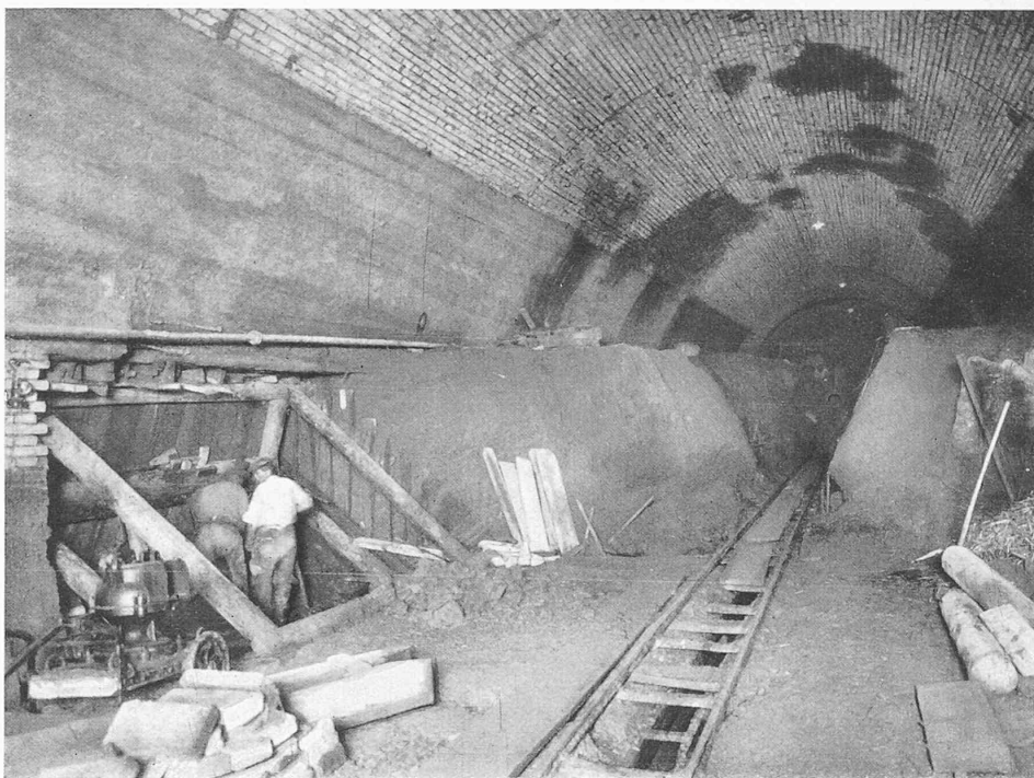
Abb. 11. Abbau der Strosse, Ausschachtung für Widerlager und Gewölbe-Unterfangung (UlMBERG).
