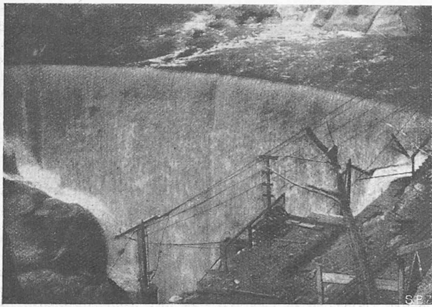
Die Versuchs-Gewölbe-Staumauer am Stevenson-Creek in Kalifornien während des Hochwassers vom 27. November 1926.
